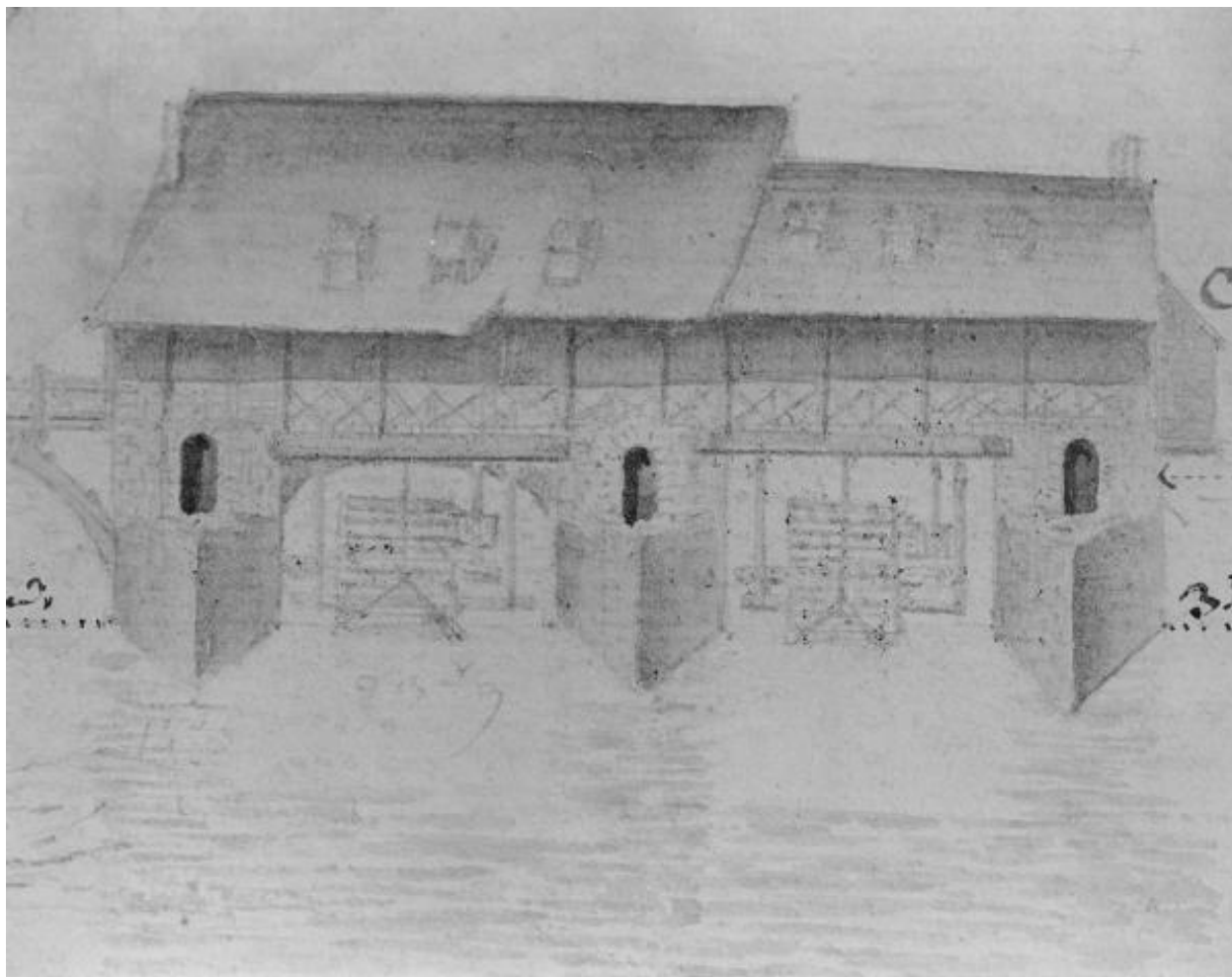
Détail, "Plan du moulin de Montjean sur la rivière de Chalennes..", dessin réhaussé à l'aquarelle par Migault, 18 septembre 1790. (AD Maine-et-Loire ; 11 Fi, carton 87, n° 454).
