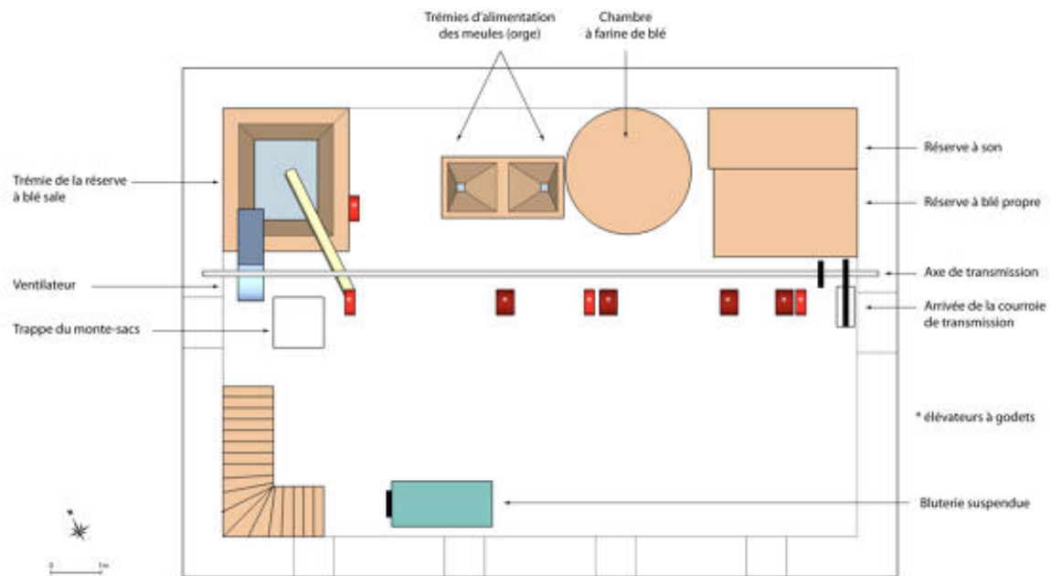
SAINT-SULPICE (53) - Moulin de la Rongère Plan schématique du deuxième étage, en partie restitué.
