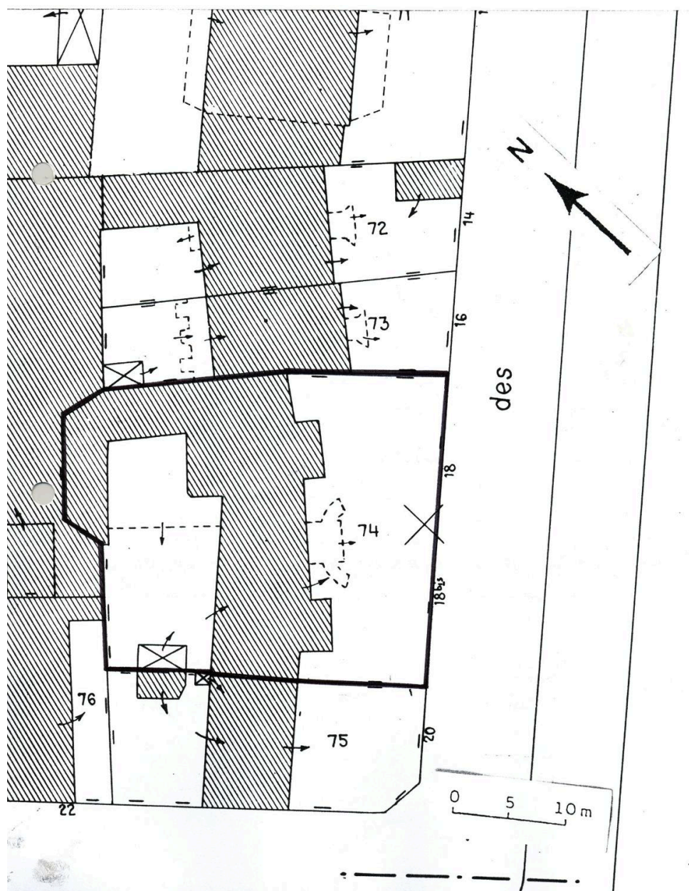
Plan-masse et de situation. D'après le plan cadastral, 1980, section HK, parcelle 74, éch. 1 : 500, agrandi.
