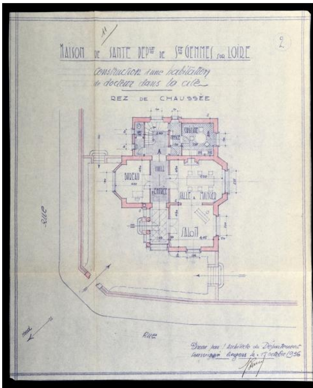
Construction d'une habitation de docteur dans la cité. Rez-de-chaussée, par Ernest Bricard. 15 octobre 1936. (Archives départementales de Maine-et-Loire, 4 N).
