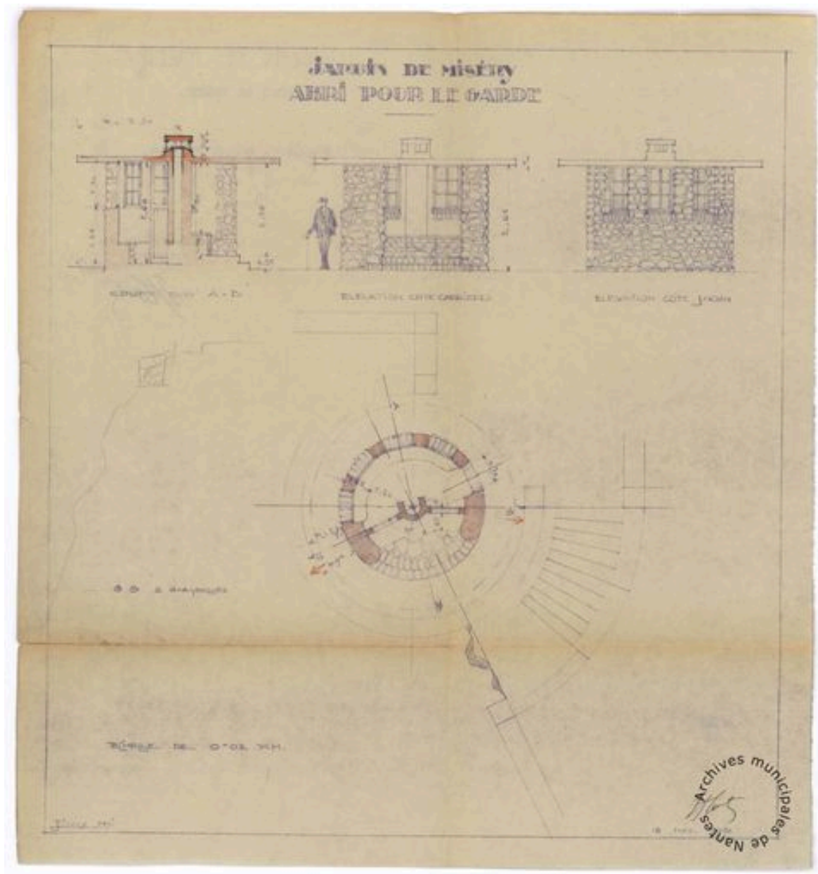
Plan de l'abri pour le garde, 1934.
