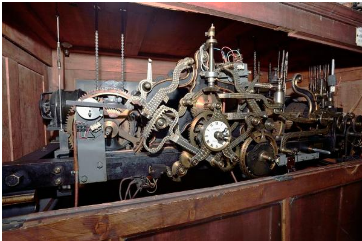
Détail du mécanisme de l'horloge.
