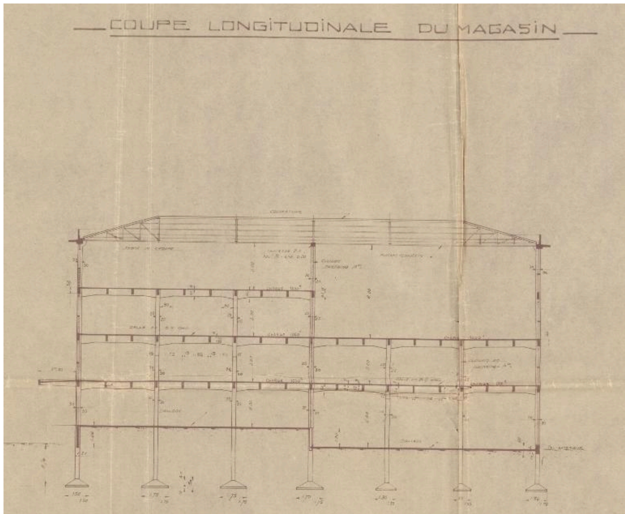
Elévation de la minoterie, 1934.
