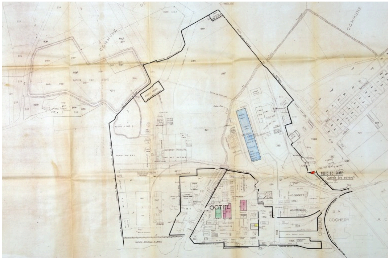
Plan général d'implantation de l'usine en 1972, détail.
