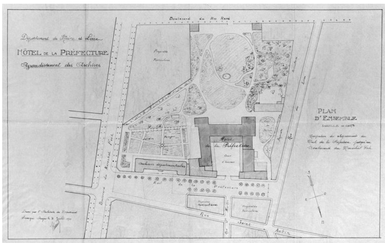
Département de Maine-et-Loire. Hôtel de la Préfecture. Agrandissement des Archives. Plan d'ensemble, par l'architecte du département Ernest Bricard, 1933. (Archives départementales de Maine-et-Loire ; 48 alpha 34).
