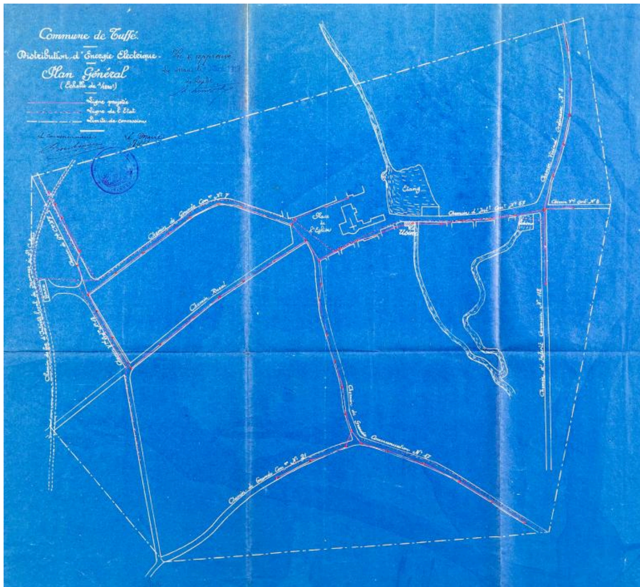
Plan du premier réseau d'électrification du bourg de Tuffé, 1913.
