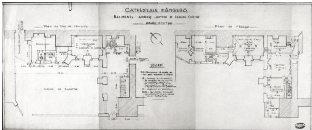
Bâtiments annexes autour de l'ancien cloître : plans du rez-de-chaussée et de l'étage. Dessin, [v. 1950], éch. 1 : 100. 27,5 x 67 cm. (Médiathèque de l'Architecture et du Patrimoine ; 55667).
