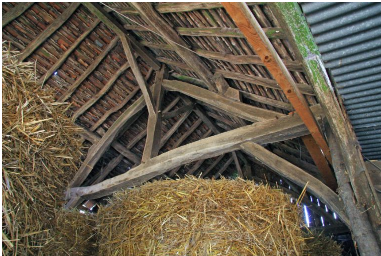
Hangar : charpente à pannes sur poteaux.
