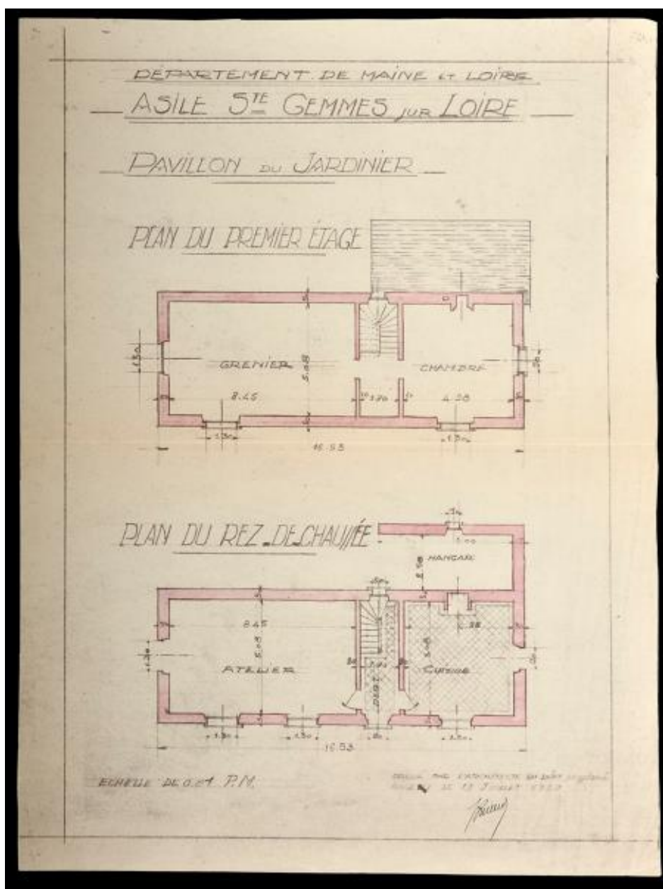
Pavillon du jardinier. Plan du premier étage et plan du rez-de-chaussée, par Ernest Bricard.19 juillet 1929. (Archives départementales de Maine-et-Loire, 4 N).
