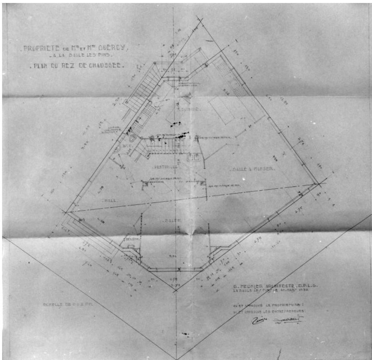
Plan du rez-de-chaussée au 1/50e de l'Atlantic Hôtel dressé par G. Meunier en 1930.
