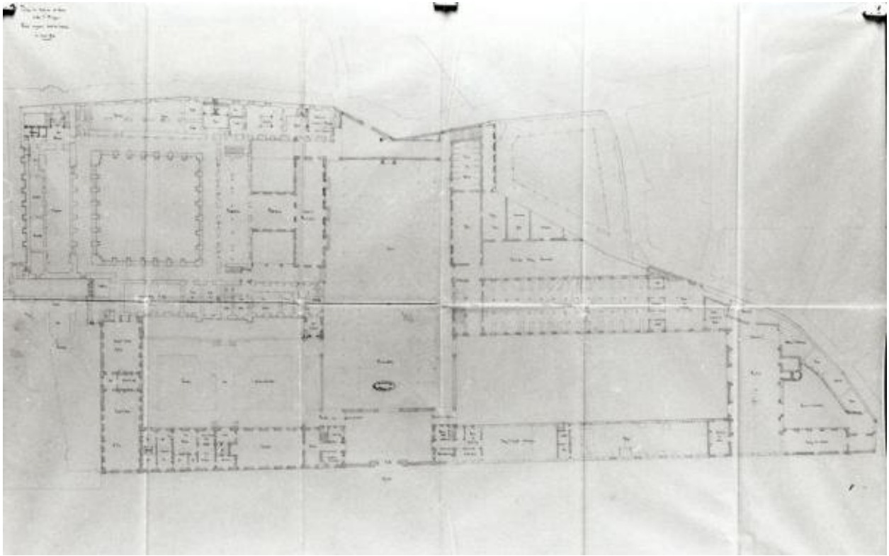
Dépt de Maine-et-Loire. Ville d'Angers, mars 1840. Programme d'agrandissement de l'école : plan au sol de l'ensemble des bâtiments.
