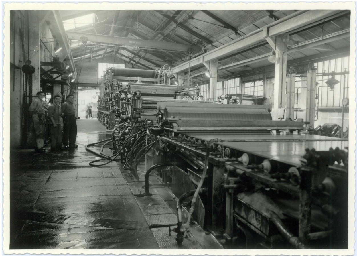
Vues de la papeterie de Bessé-sur-Braye au XXe siècle. Vue de la machine à papier 1, arrêtée en 1964, dans le 1er atelier de fabrication de la papeterie (bâtiment A2).
