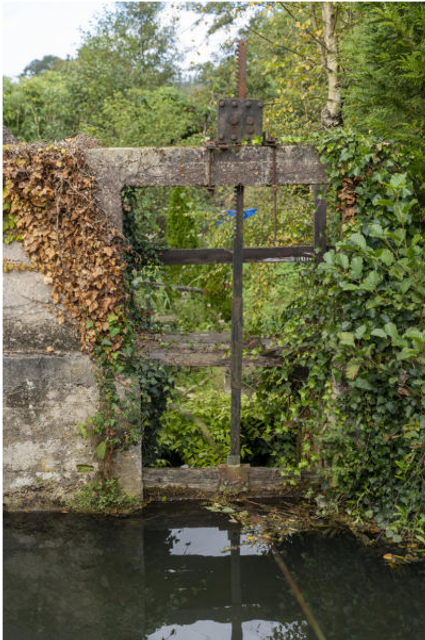
Vanne de décharge du moulin de Cherruau.
