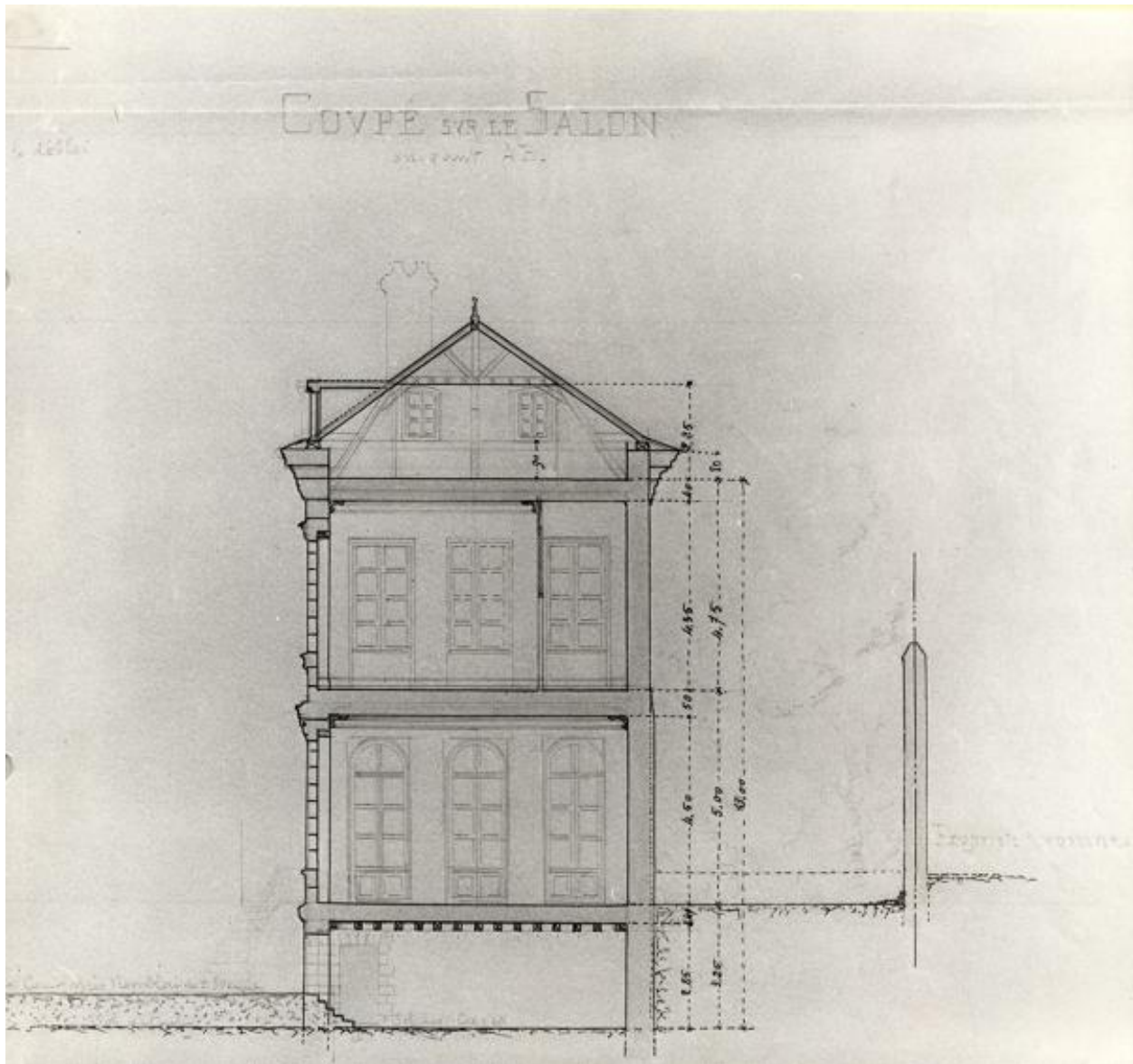
Elévation transversale gauche, projet, par l'architecte Auguste Martin. Dessin, fin 19e siècle, éch. 1:100e. (Collection particulière, M. Pousset).
