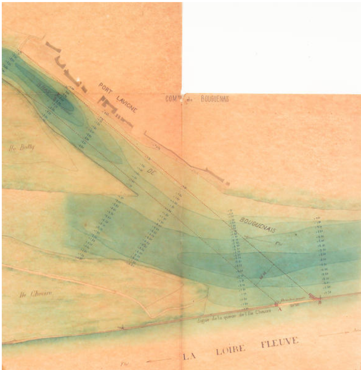
Plan joint au projet d'amélioration du bras de Bouguenais en face de Port-Lavigne, 1872.
