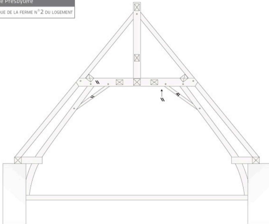
Élévation schématique de la ferme n° 2 de la charpente du logement.
