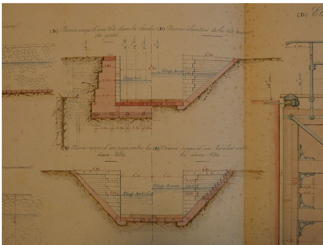
Projet de reconstruction du barrage éclusé, par l'ingénieur Espitallier, 1867 : coupes de l'écluse.
