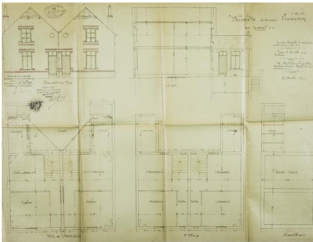
Plan, coupe et élévation d'une maison rue Joubert.
