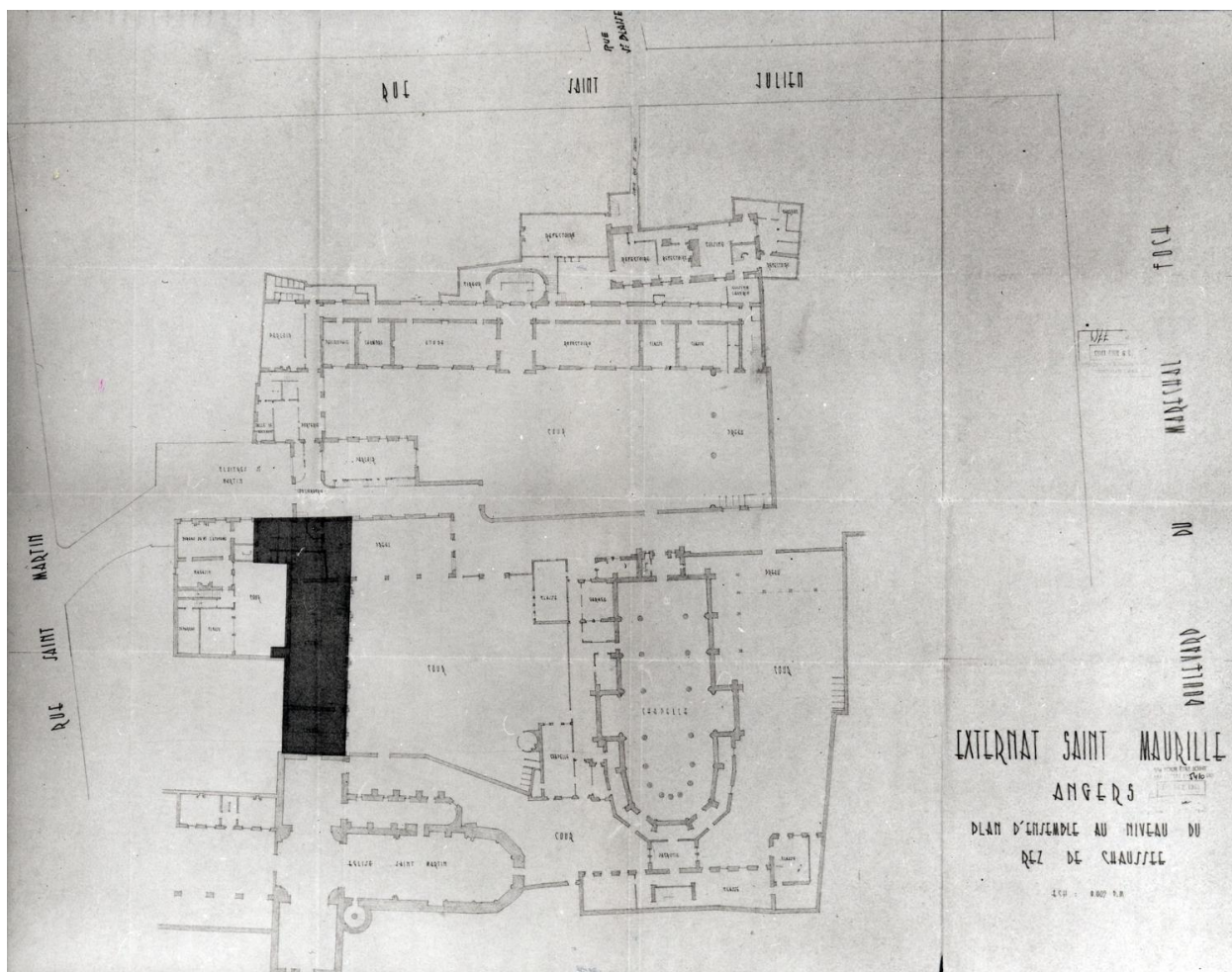
Plan général du rez-de-chaussée de l'établissement scolaire, par A. Monet et J. Samain, 1955. En sombre, le bâtiment de classes faisant l'objet d'une surélévation.
