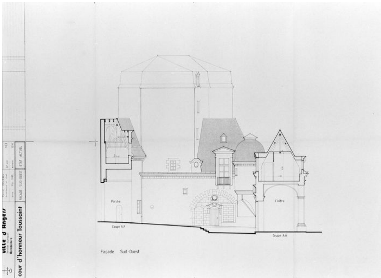
Cour d'honneur Toussaint. Façade sud-ouest. Etat actuel, relevé, visé par D. Roussel, architecte en chef de la Ville d'Angers, 1985. (Ville d'Angers, service architecture ; dossier 8502).
