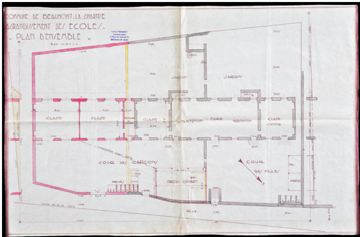
Plan d'ensemble pour l'agrandissement des écoles.
