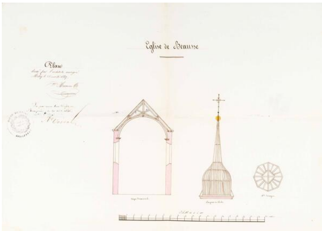
Église paroissiale de Beausse. Coupe et clocher dressés par François Humeau, architecte, le 25 mars 1847. (AM Beausse ; 1 M 5).
