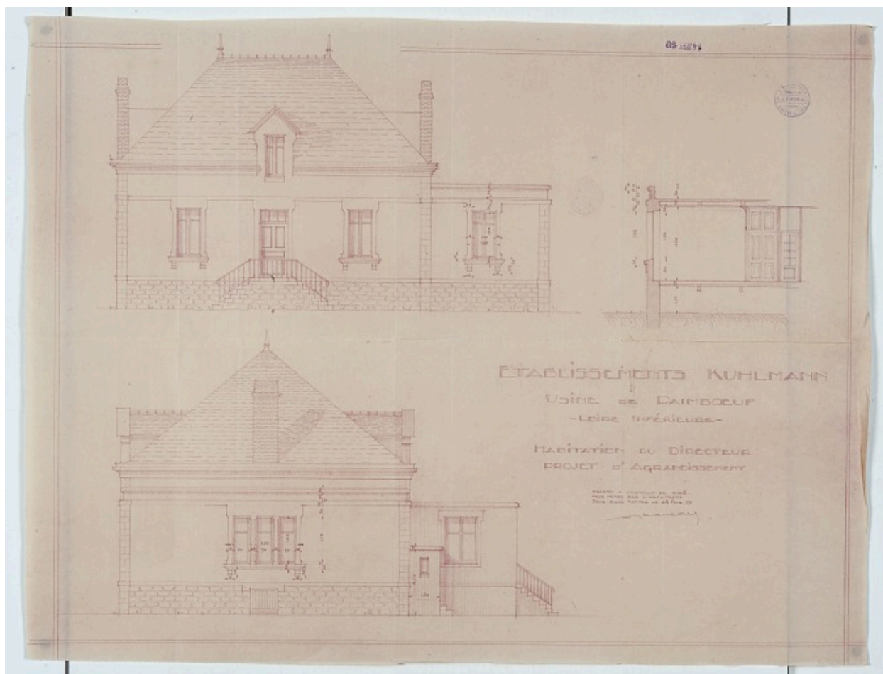
Élévation projetée du côté de la façade ouest, A.-J. Daveau (architecte), 1929.
