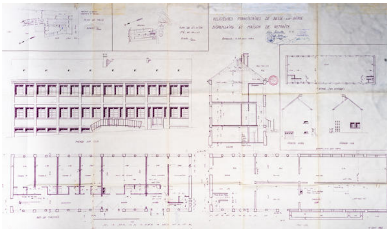
Plan, coupe et élévation du dispensaire et maison de retraite.
