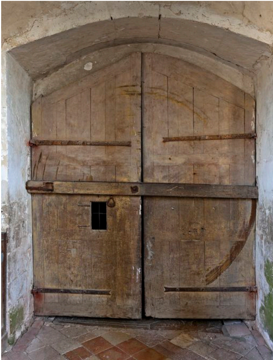
Revers des vantaux avec barre de fermeture pivotante en position fermée.
