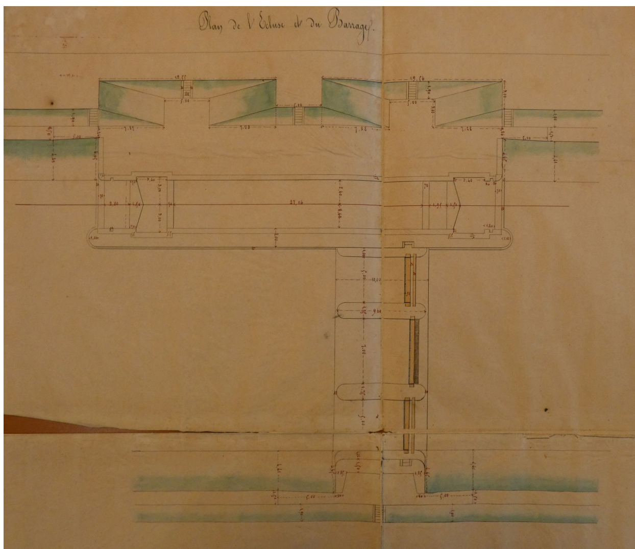
Projet de barrage éclusé sur la Vieille Sèvre par Joseph Maire, 1855 : plan.
