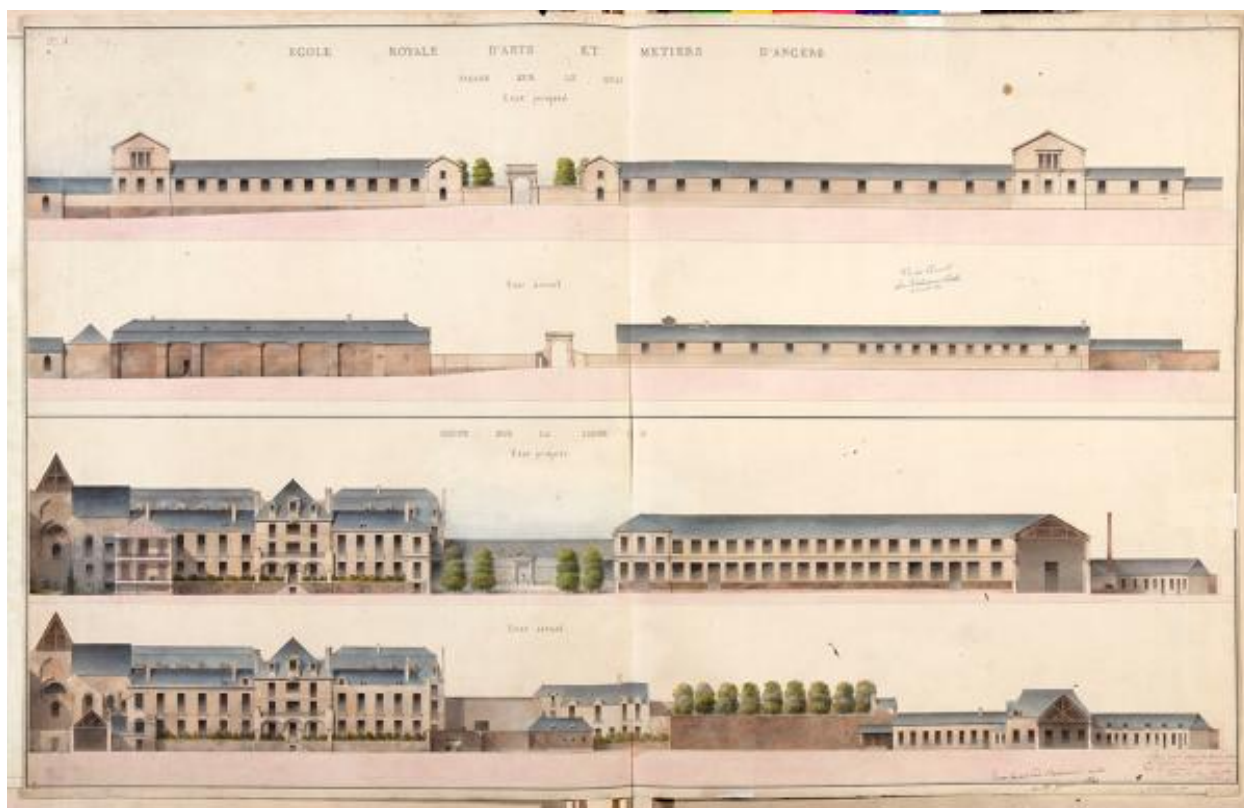
Ecole royale des Arts-et-Métiers. Façade sur le quai. Coupe sur la ligne CD [sud-nord le long de l'aile Est du cloître et du bâtiment d'ajustage]. A gauche, les l'église et les bâtiments conventuels. Etat projeté. Etat actuel, par Ch.-E. Isabelle, 1839.
