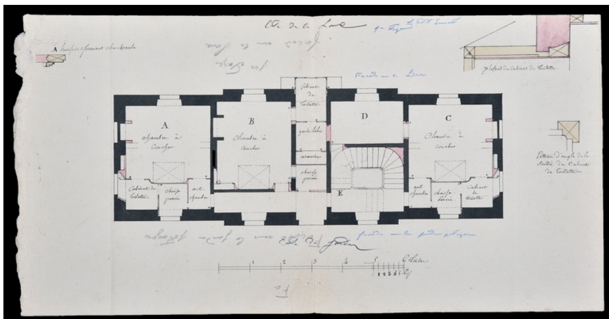
Plan du 1er étage. Vers 1808. (Archives départementales de Maine-et-Loire, 103 J 33/15).
