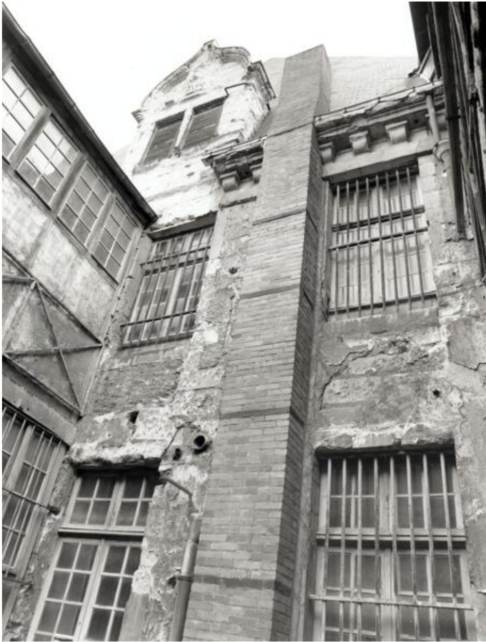
Aile sud du cloître : élévation ouest sur une courette enclavée (le long de la rue de la Censerie). A gauche, constructions adventices.
