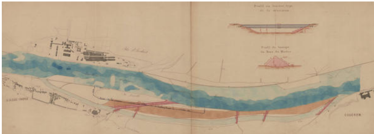
Plan de dérivation du bras du Mastro, 1895.
