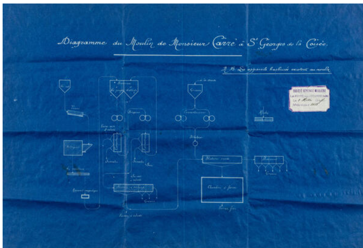
Diagramme schématique du circuit de production, 1907.
