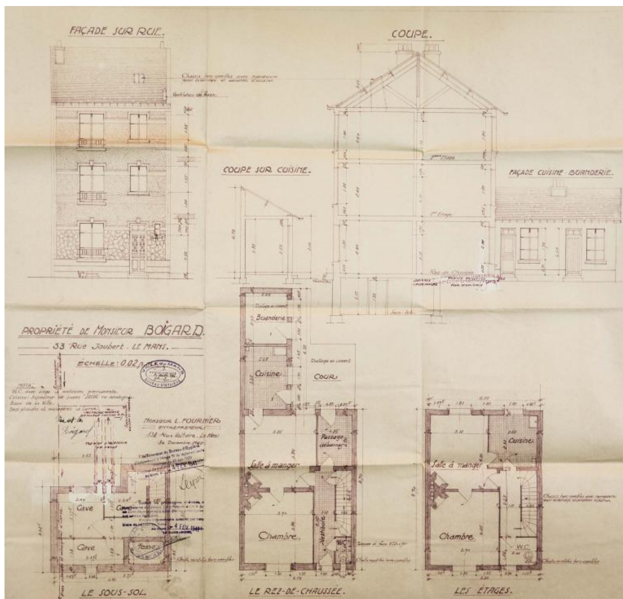
Plan, coupe et élévation d'un immeuble rue Joubert.
