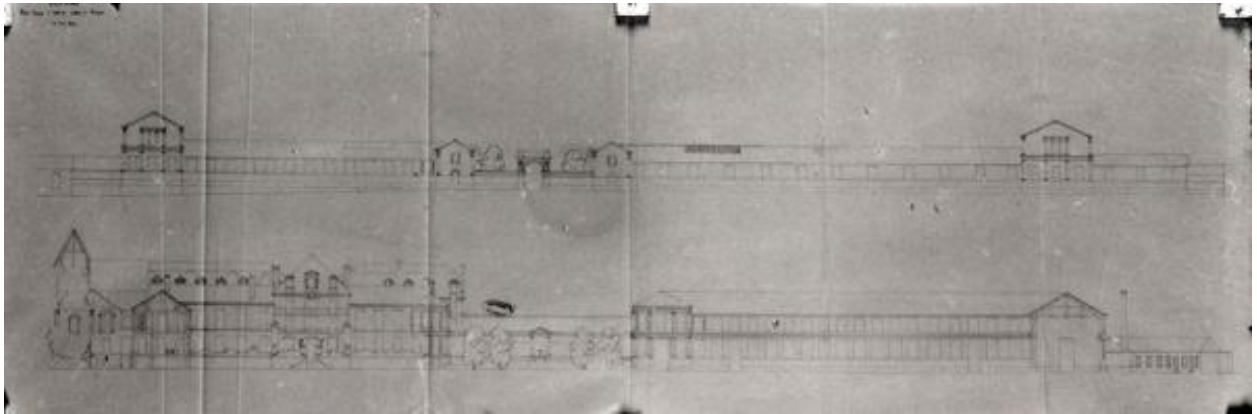
Maine-et-Loire. Ecole royale d'arts et métiers à Angers, vu mai 1842. Programme d'agrandissement de l'école. Deux élévations : en haut sur la rue du Godet et en bas, à hauteur du logis abbatial.
