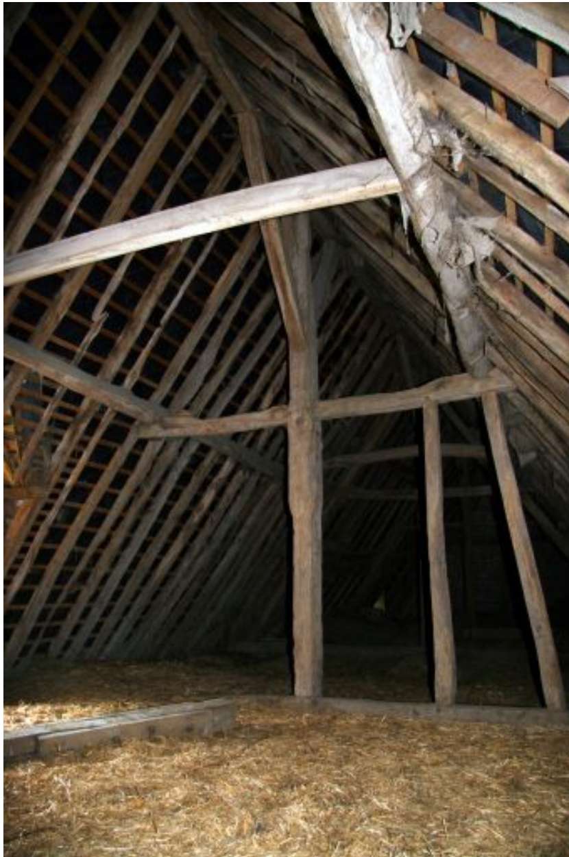
La grange : charpente à pannes.
