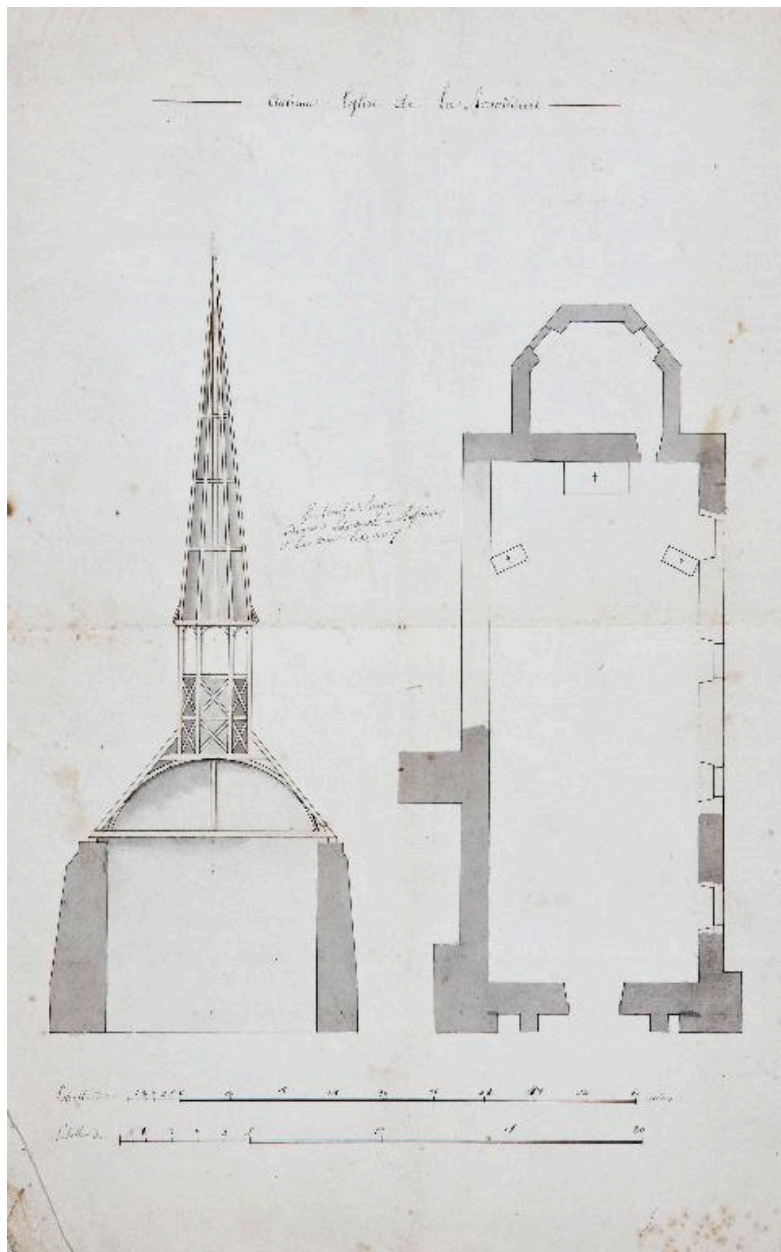
Plan et coupe transversale de l'ancienne église.
