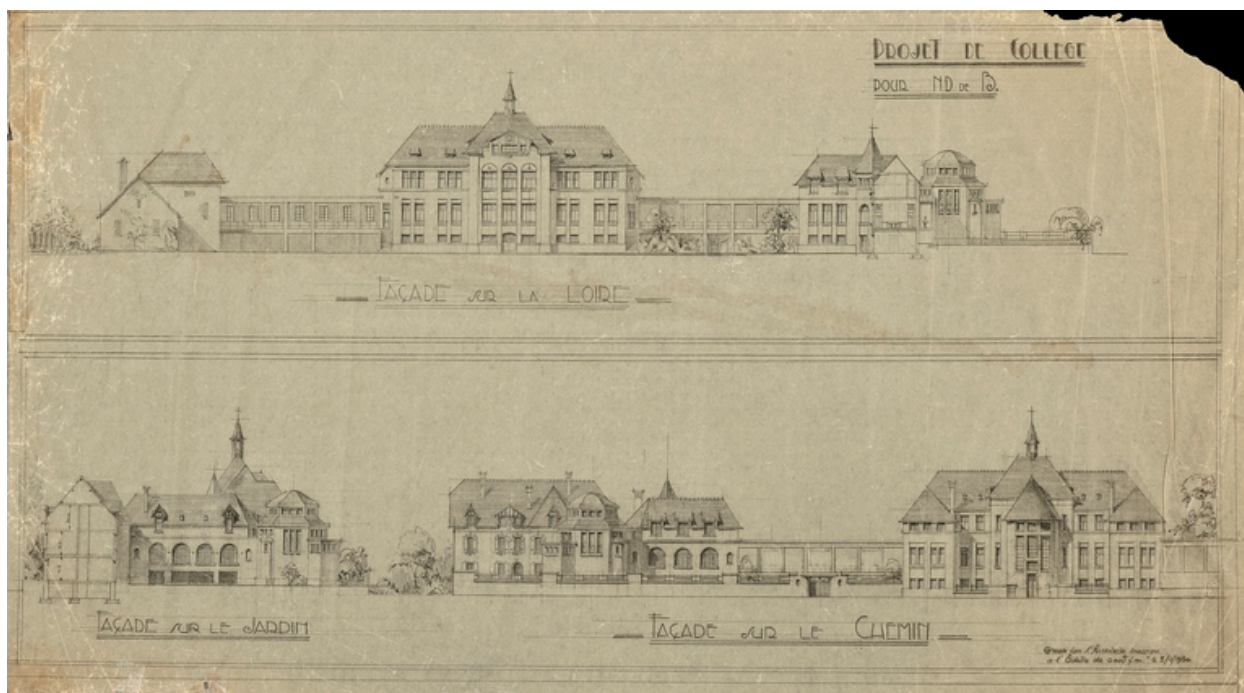
Projet de collège pour Notre-Dame de Béhuard. Façade sur la Loire. Façade sur le jardin. Façade sur le chemin. n.s., le 3 février 1930.
