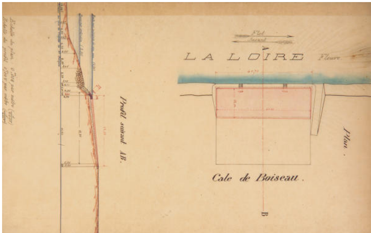
Cale de Boiseau. Exhaussement du tablier. Plan et profil.
