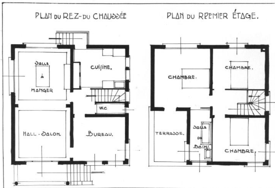
VILLA MODERNE — M. RENÉ PERREY, ARCHITECTE D. P. L. G.
