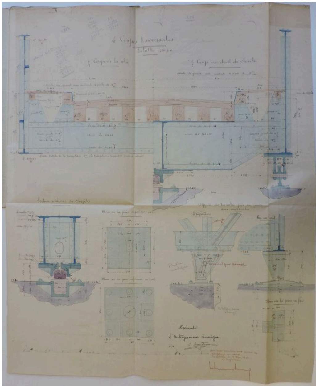
Coupe transversale de la travée tournante métallique, par l'entrepreneur Jaudeau, 1913.
