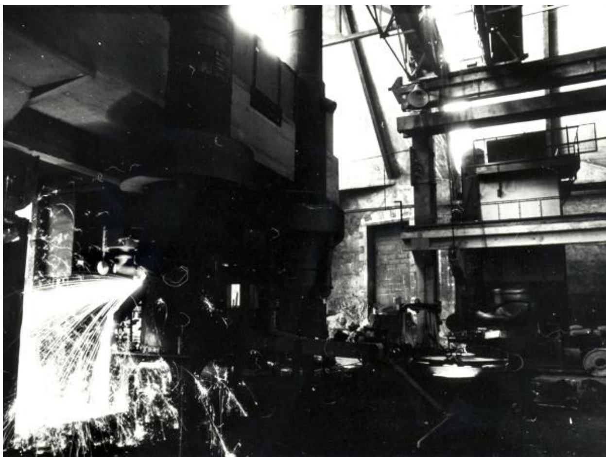
Atelier de fonderie : cubilot gauche. Ecoulement du laitier.
