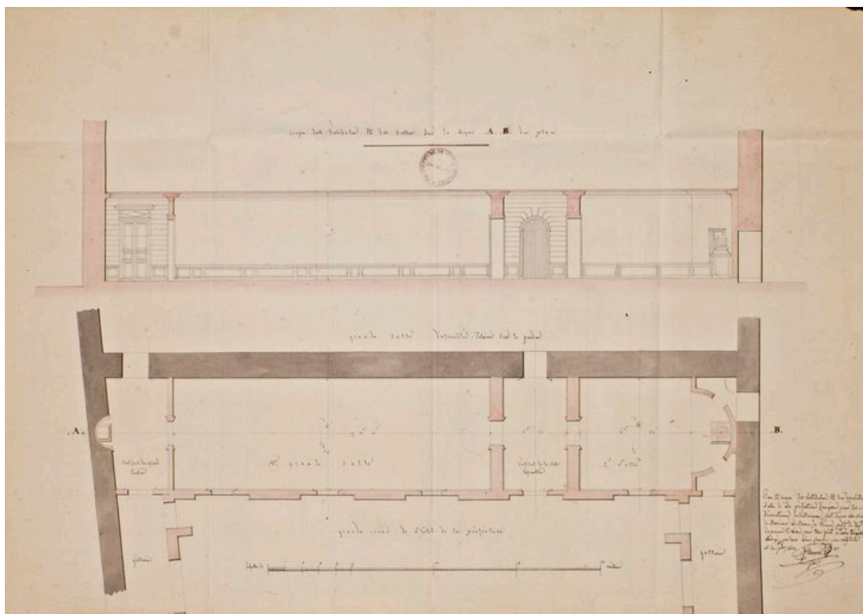
Plan et coupe des vestibules et des nouvelles salles de la préfecture d'Angers pour les décorations de l'intérieur... pour être joint au devis estimatif rédigé par nous L. François, 1821. (Archives départementales de Maine-et-Loire ; N 1766).
