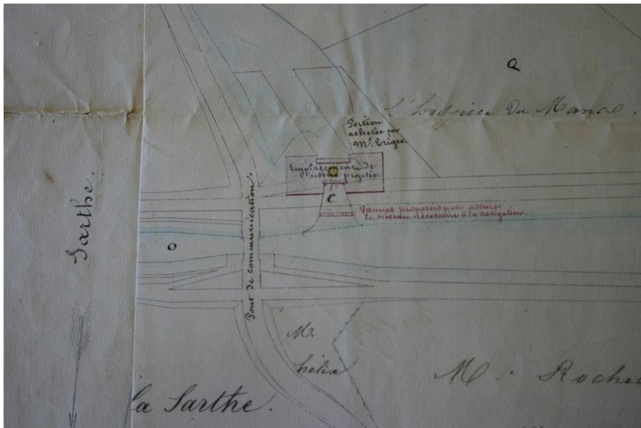
Plan de la minoterie et de ses installations hydrauliques.
