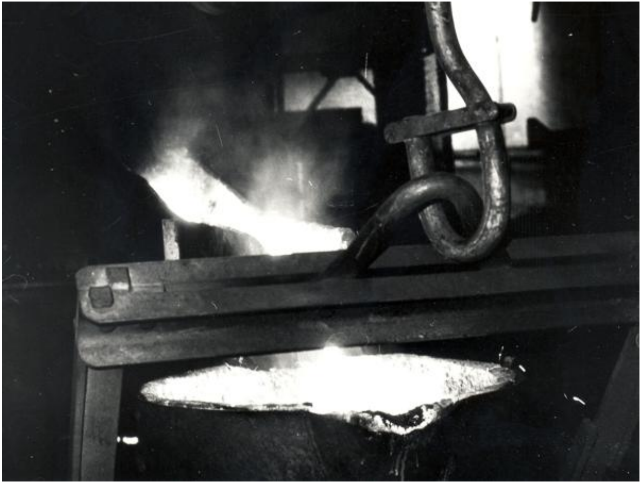
Atelier de fonderie, coulée de la fonte dans le creuset.
