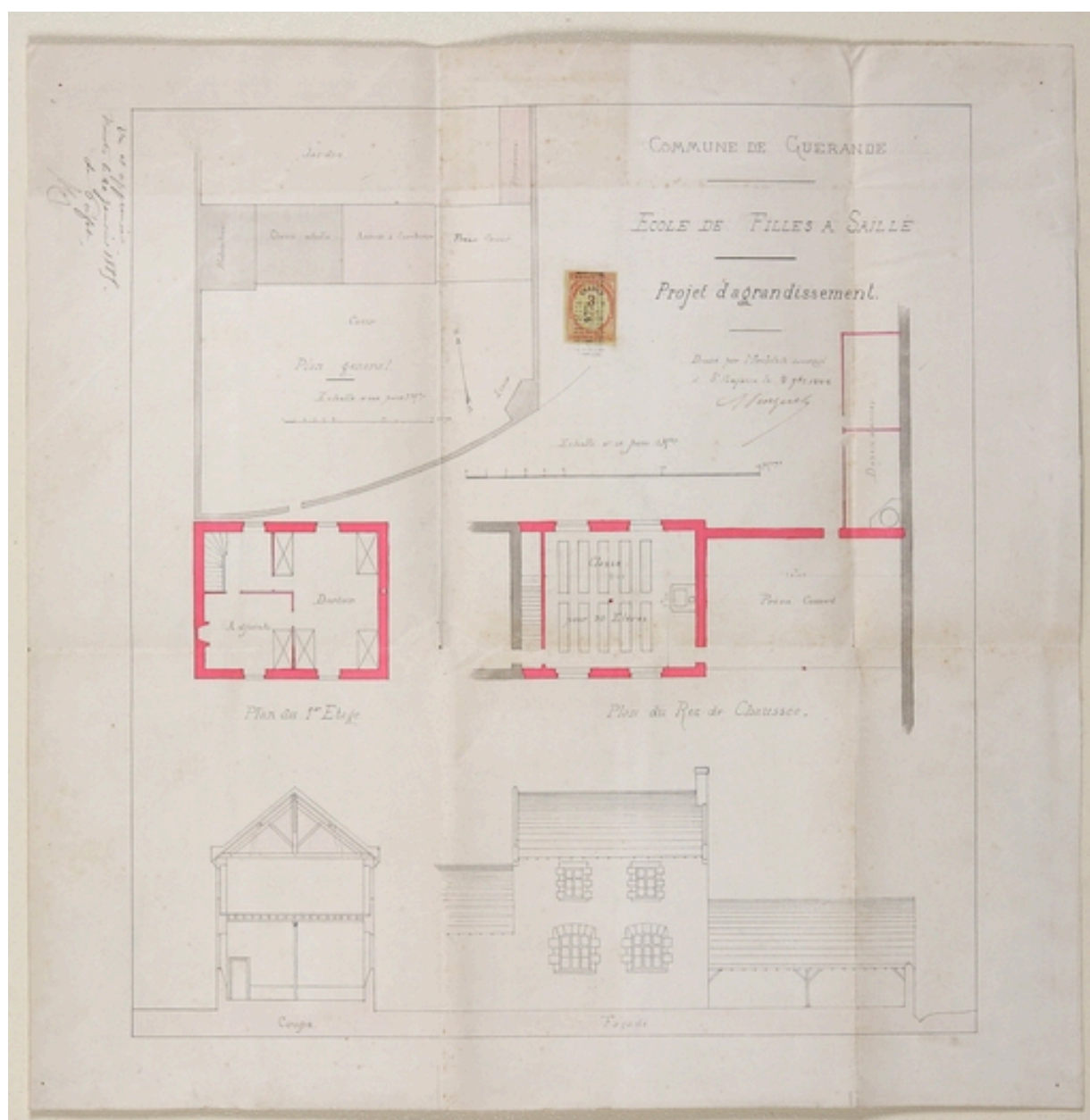
Projet d'agrandissement de l'école publique des filles de Saillé, dressé par A. Pinguet (1882).
