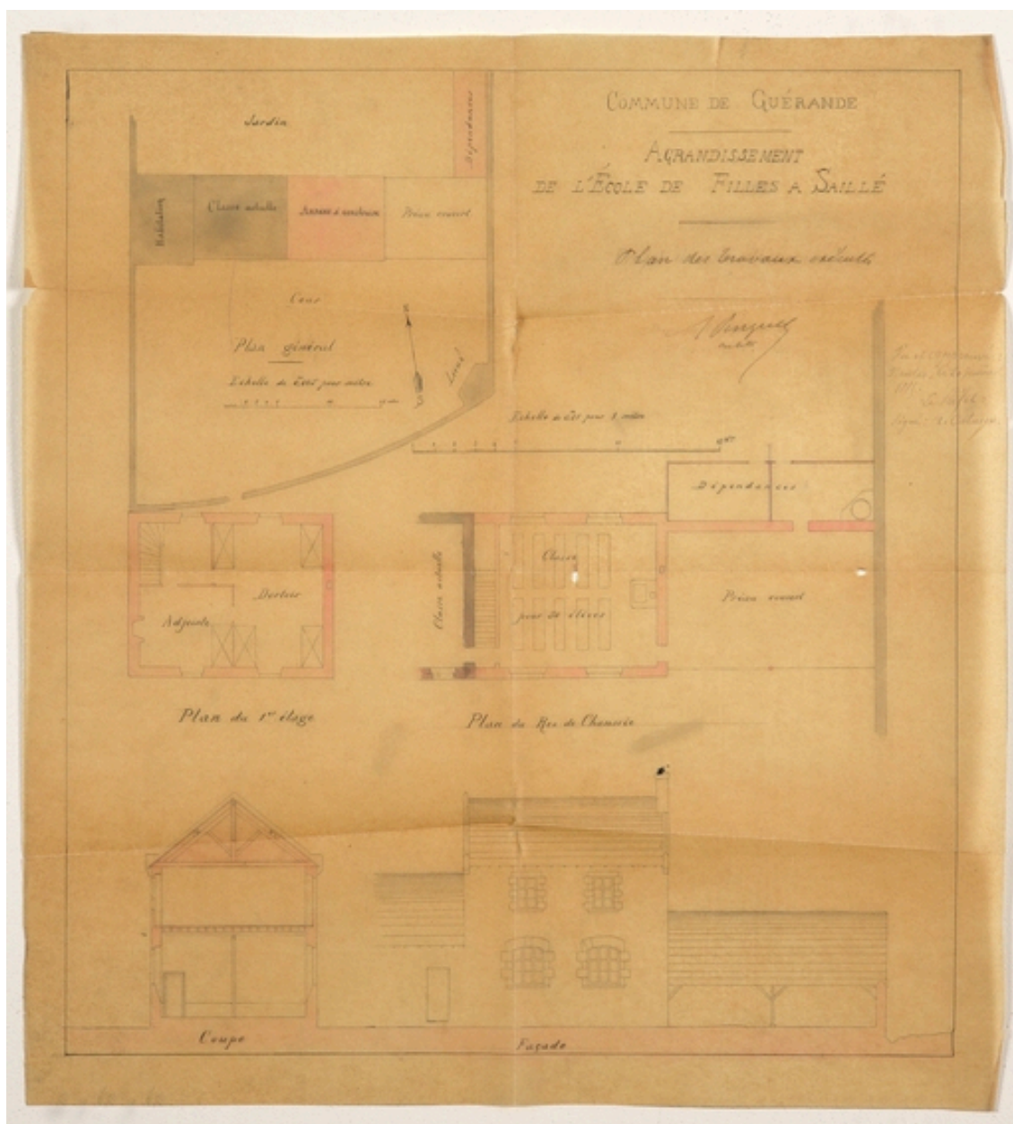
Plan des travaux exécutés en 1886 par A. Pinguet.
