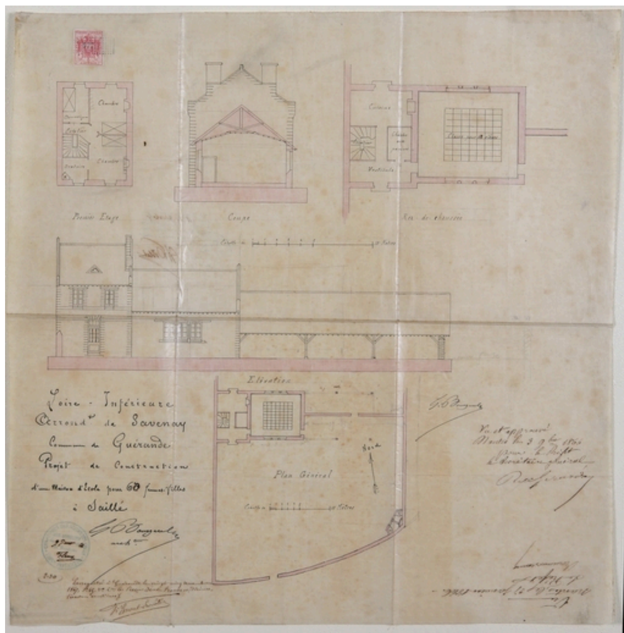
Deuxième projet de construction d'une école publique de fille à Saillé, dressé par G. Bourgenel (1866).
