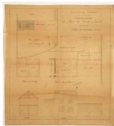
Plan des travaux exécutés en 1886 par A. Pinguet. Autr. Auguste Pinguet, Phot. Denis (reproduction) Pillet IVR52_20084400419NUCA
