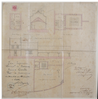
Deuxième projet de construction d'une école publique de fille à Saillé, dressé par G. Bourgenel (1866). Autr. Gustave Bourgerel, Phot. Denis (reproduction) Pillet IVR52_20084400422NUCA
