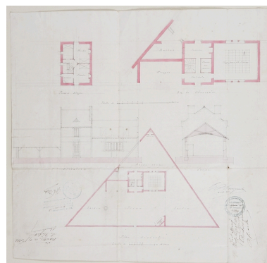
Premier projet pour la construction de l'école de filles de Saillé sur un terrain appartenant à M. Million, dressé par G. Bourgenel (1866). Autr. Gustave Bourgenel, Phot. Denis (reproduction) Pillet IVR52_20084400415NUCA
