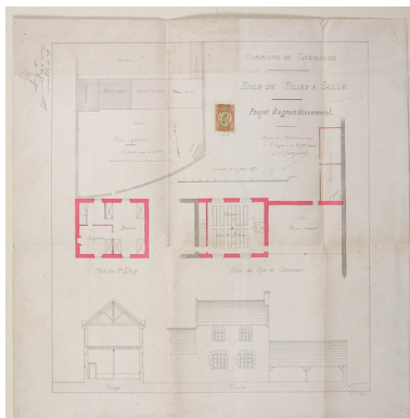
Projet d'agrandissement de l'école publique des filles de Saillé, dressé par A. Pinguet (1882). Autr. Auguste Pinguet, Phot. Denis (reproduction) Pillet IVR52_20084400421NUCA
