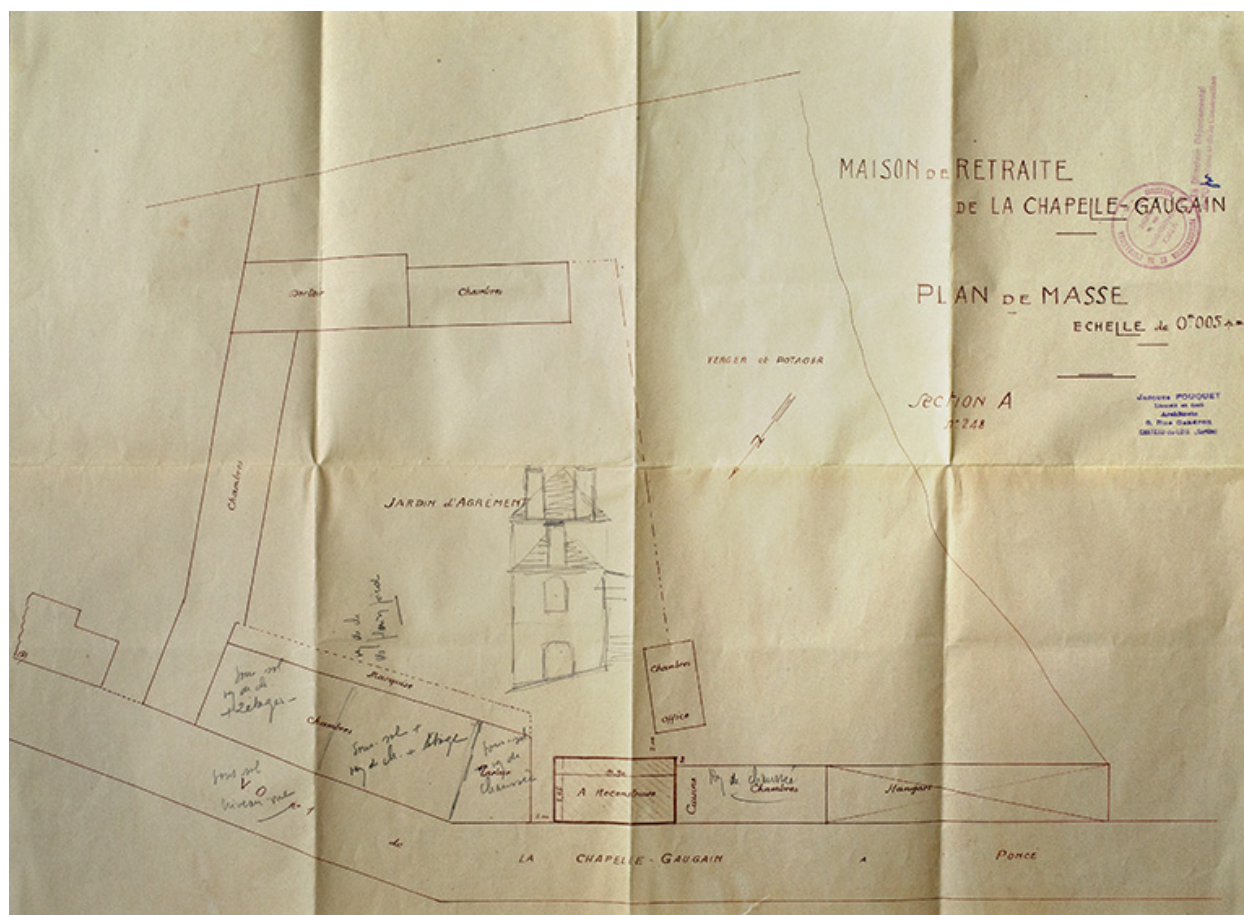
Plan masse du couvent, vers 1958, Jacques Fouquet architecte.
