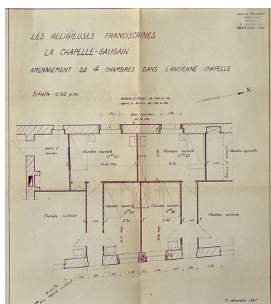
Projet d'aménagement de quatre chambres dans l'ancienne chapelle [oratoire], 16 décembre 1961, Jacques Fouquet architecte. Autr. Jacques Fouquet, Phot. Pierre-Bernard Fourny IVR52_20147200068NUCA
