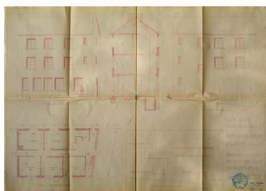
Bâtiment neuf sur le VO1, projet de construction d'un 2e étage, vers 1961, Jacques Fouquet architecte.
