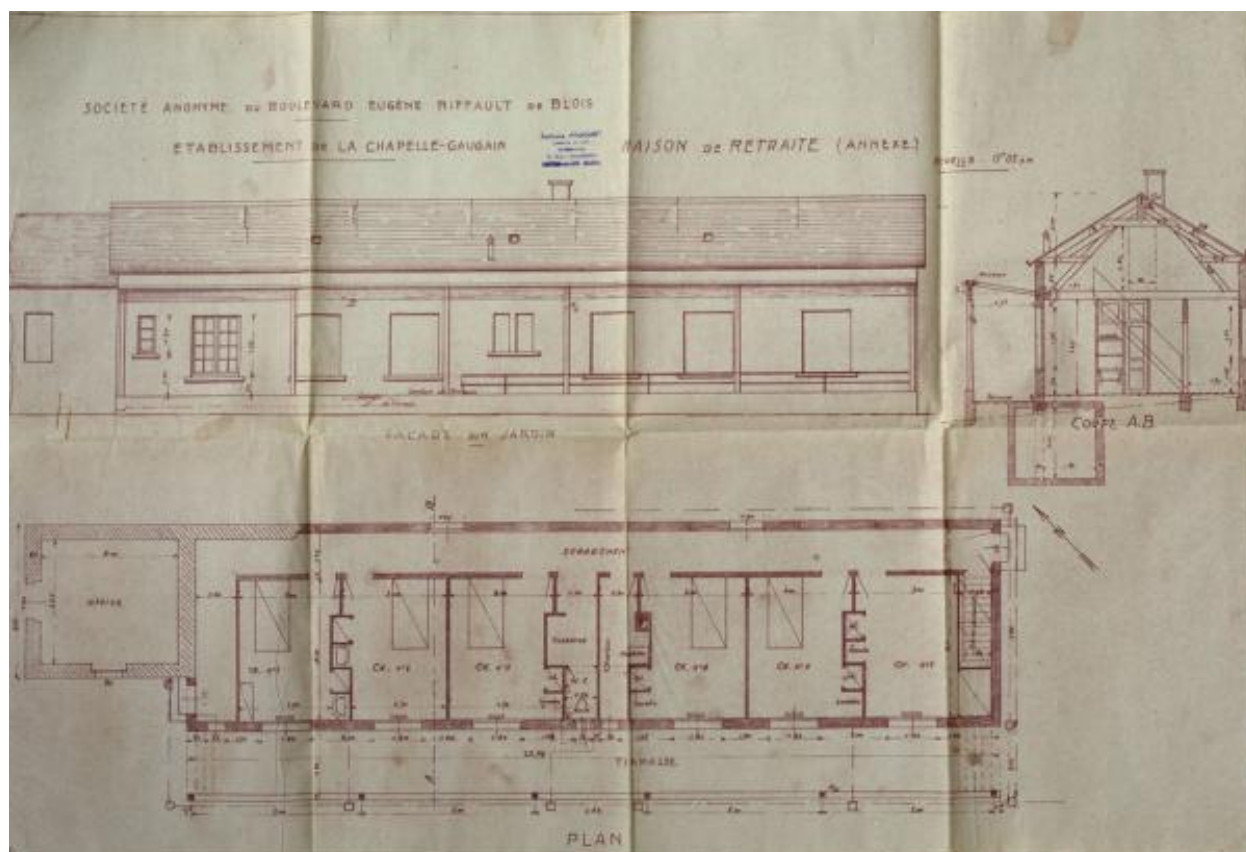
Maison de retraite en rez-de-chaussée (annexe), Jacques Fouquet architecte.
