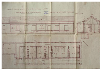
Maison de retraite en rez-de-chaussée (annexe), Jacques Fouquet architecte. Phot. Pierre-Bernard Fourny, Autr. Jacques Fouquet IVR52_20147200069NUCA
