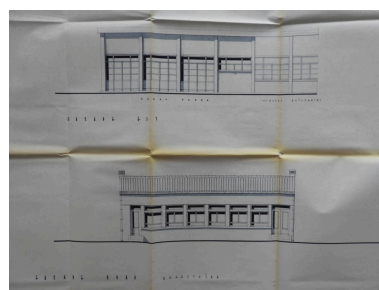
Projet de préau prolongeant le collège (en haut) et de cuisine-réfectoire au sud de la cour, par Jean Salmas, avril 1964. Phot. Yannis (reproduction) Suire IVR52_20198500939NUCA
