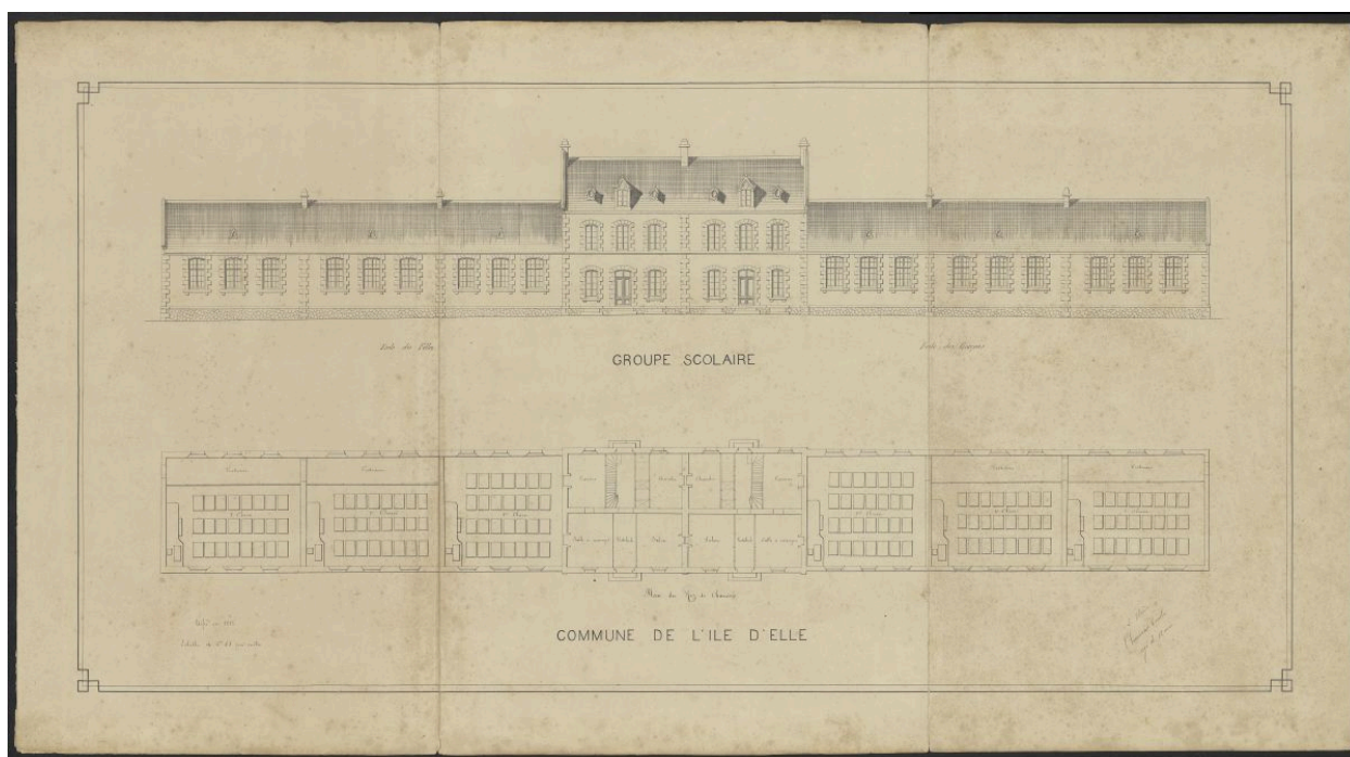
Plan et élévation du groupe scolaire réalisé en 1890 par l'élève Emile Chauveau, extrait de l'Atlas scolaire de L'Île-d'Elle.
