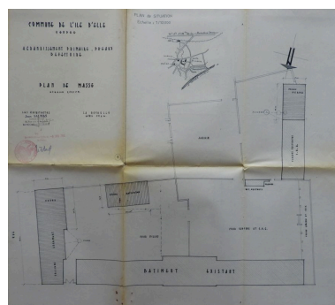
Projet d'agrandissement de l'école par Jean Salmas, avril 1964 : plan masse. Phot. Yannis (reproduction) Suire IVR52_20198500940NUCA
