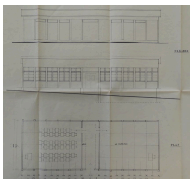
Projet de collège par Jean-Baptiste Durand en 1960 : élévations et plan. Phot. Yannis (reproduction) Suire IVR52_20198500921NUCA
