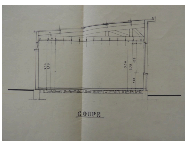
Projet de collège par Jean-Baptiste Durand en 1960 : coupe. Phot. Yannis (reproduction) Suire IVR52_20198500922NUCA
