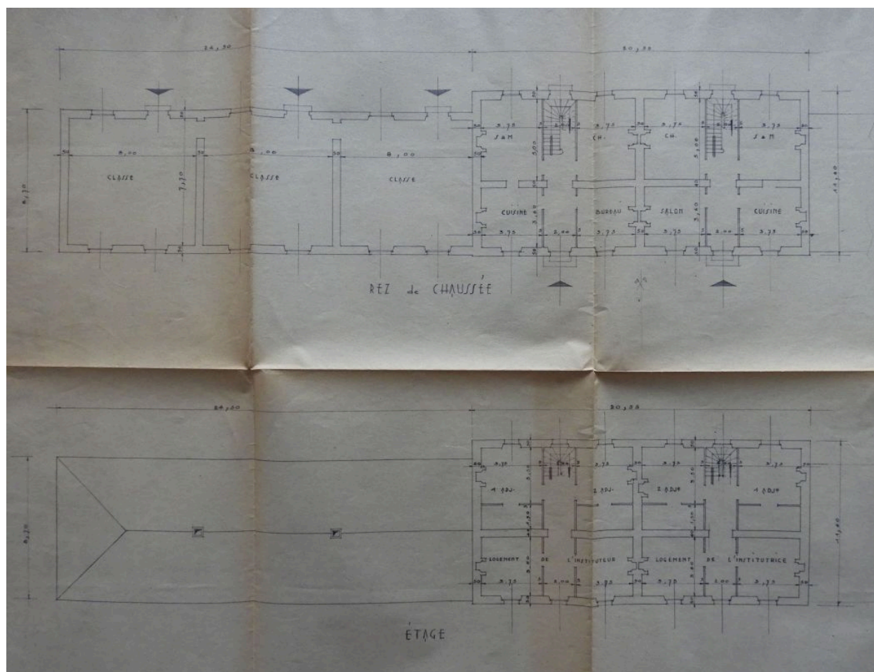
Plan du bâtiment central (logements de fonction) et de l'aile ouest par Jean-Baptiste Durand en 1956.
