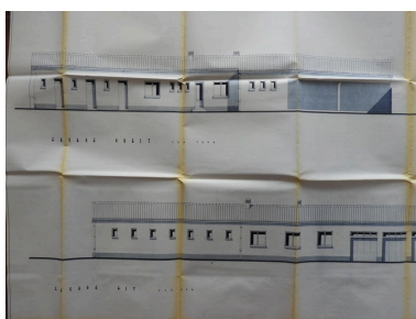
Projet de celliers, logement de fonction et préau par Jean Salmas, avril 1964 : élévations. Phot. Yannis (reproduction) Suire IVR52_20198500941NUCA
